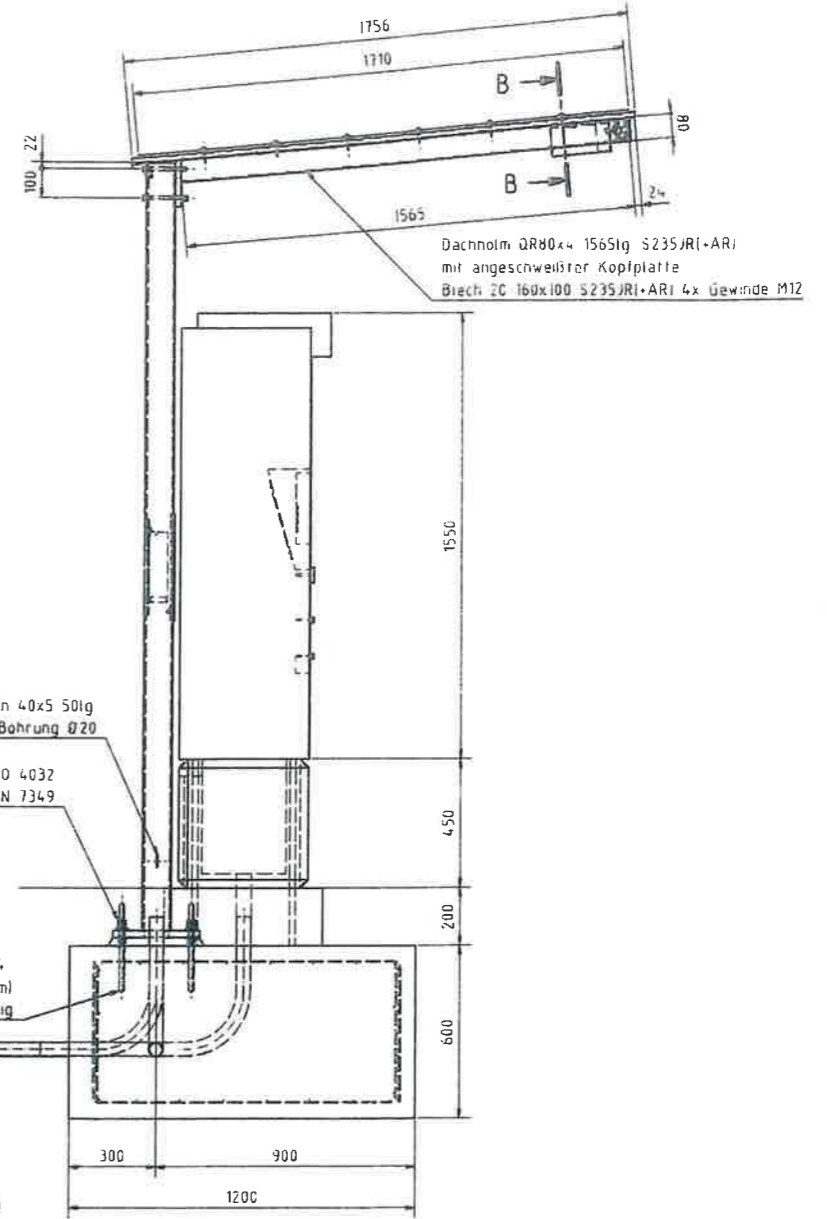
Seitenansicht ( 1 : 12,5 )
