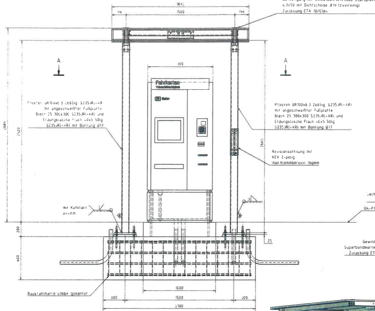
Vorderansicht ( 1 : 12,5 )
