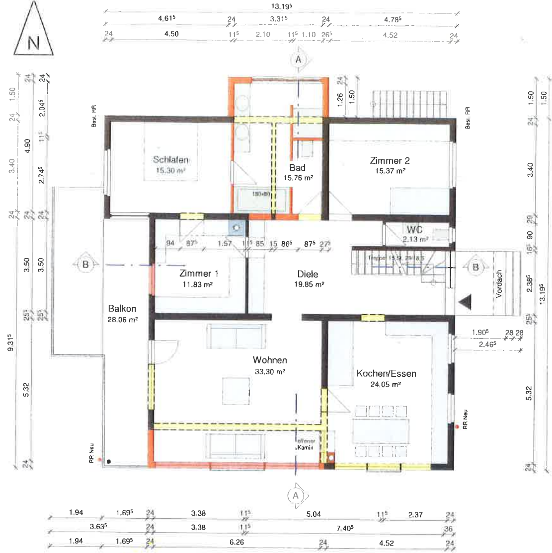
Erdgeschoss
