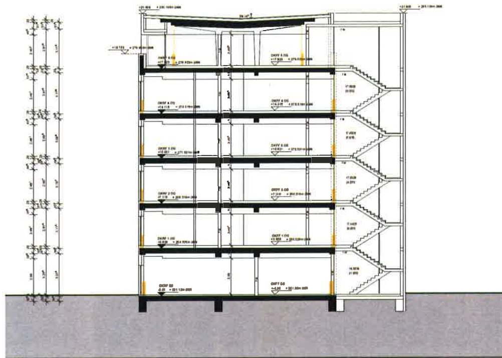
SCHNITT A-A
