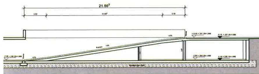
SCHNITT C-C
