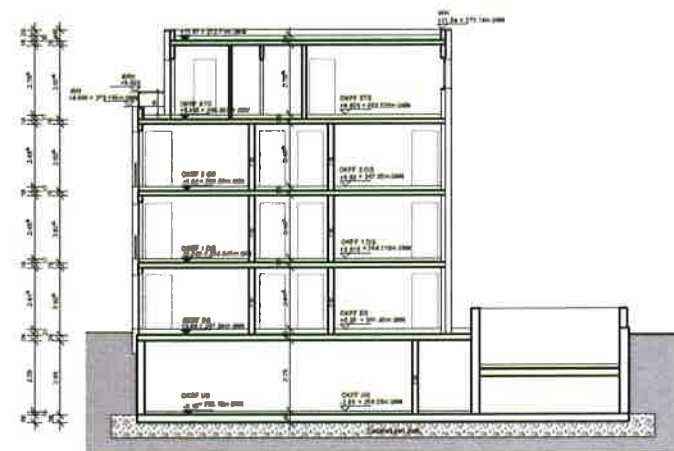
SCHNITT B-B
