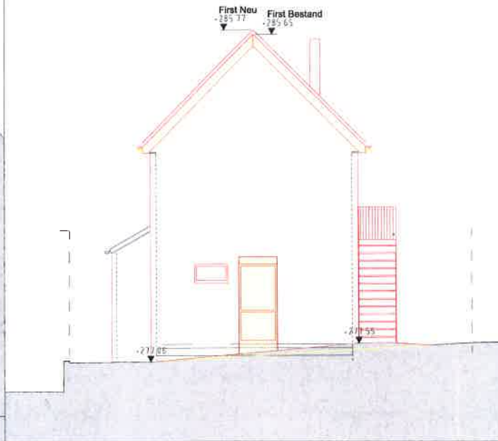
Ansicht Nord
