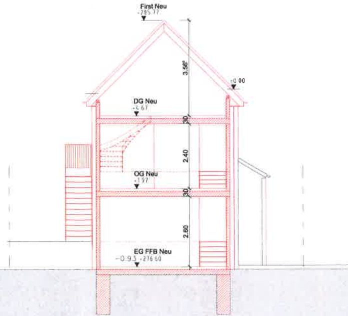
Schnitt B-B
