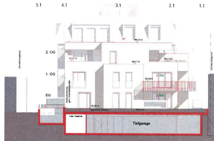
ANSICHT WEST HAUS 2
