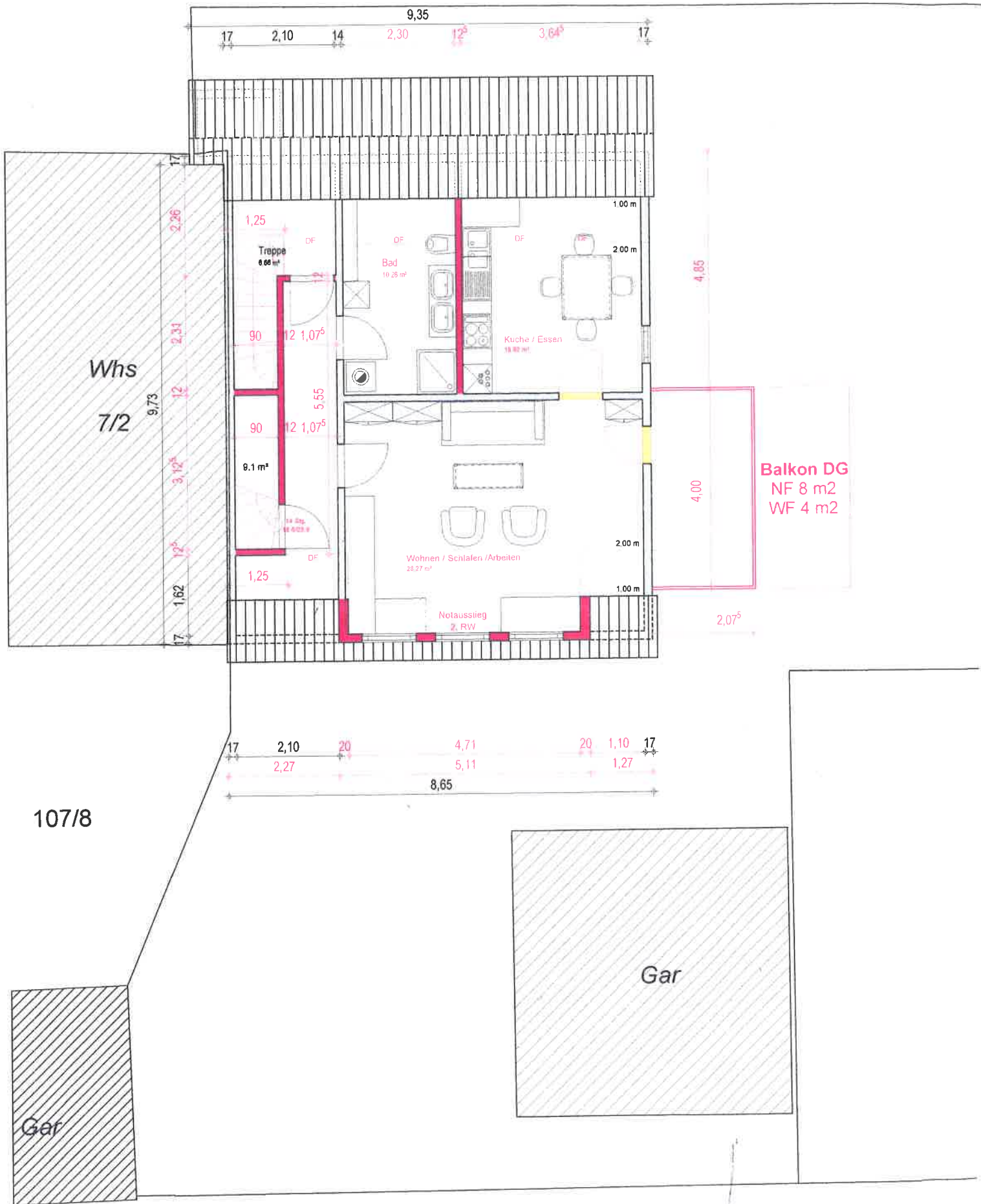
Grundriss DG v. 11.05.2020 M 1:100
