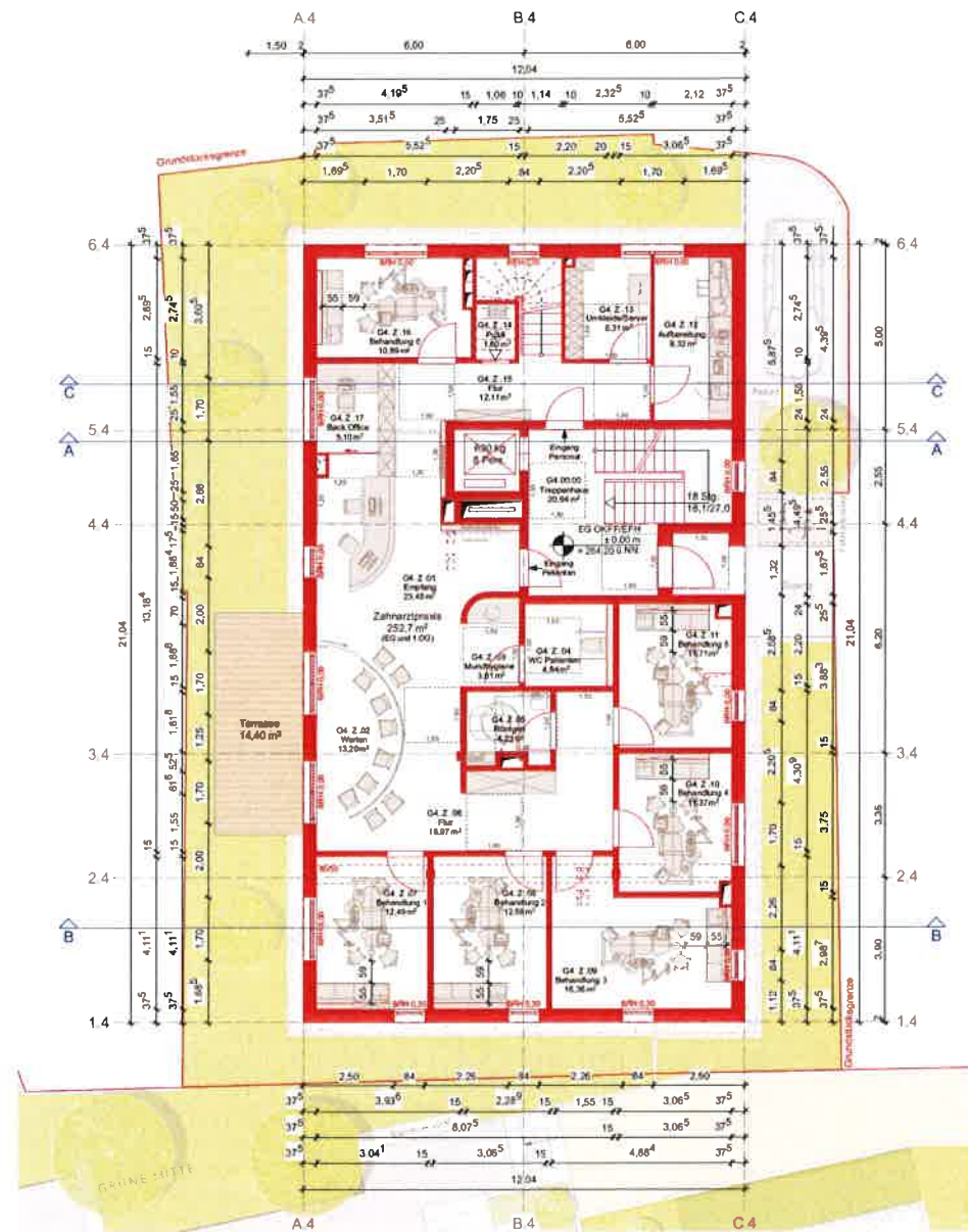
Grundriss Erdgeschoss
