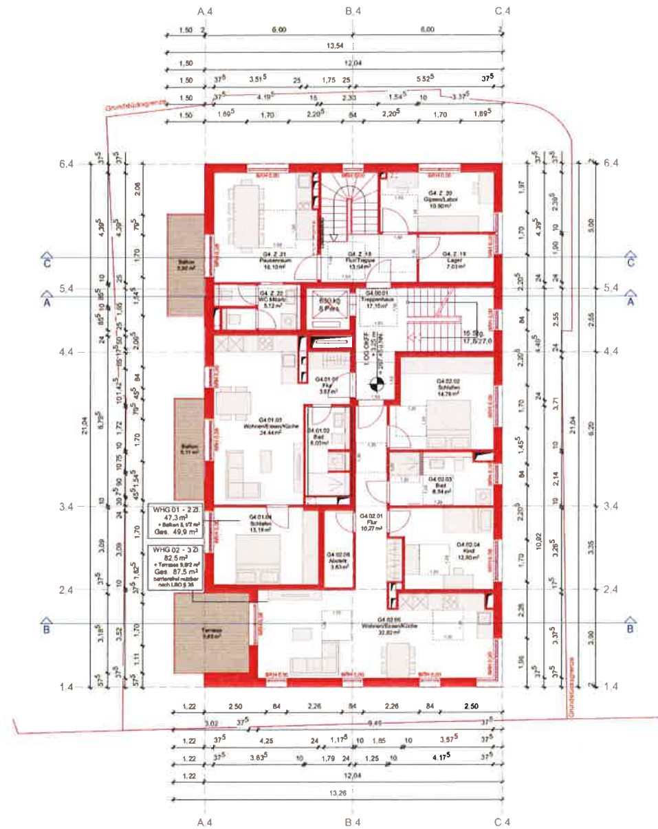
Grundriss 1. Obergeschoss
