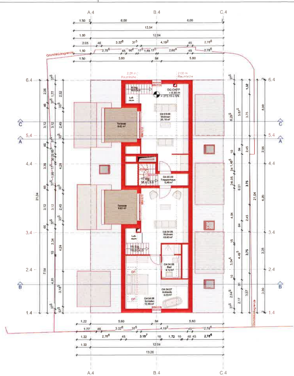
Grundriss Dachgeschoss
