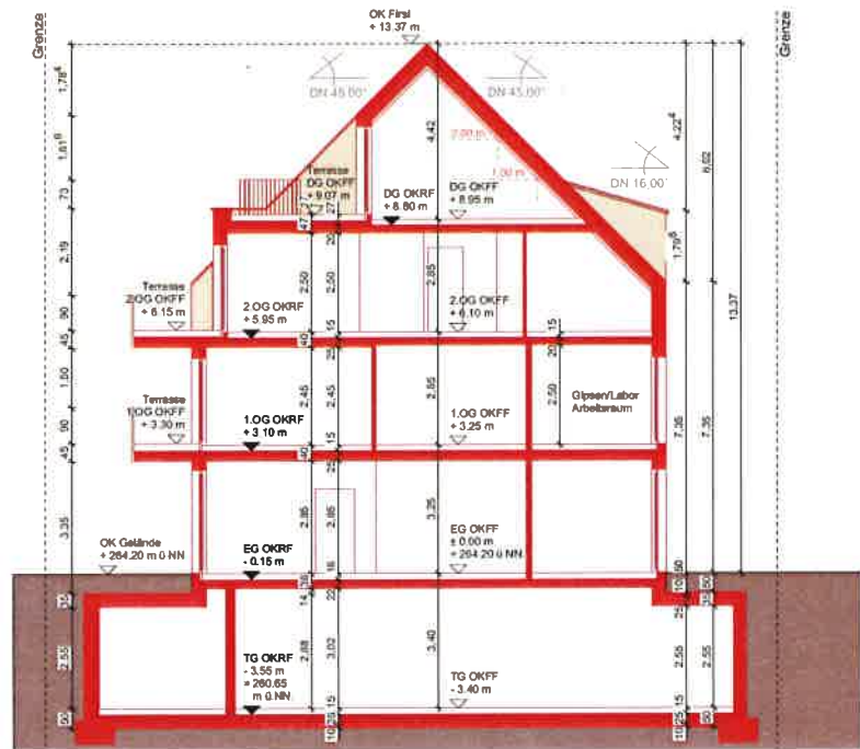
Schnitt C-C
