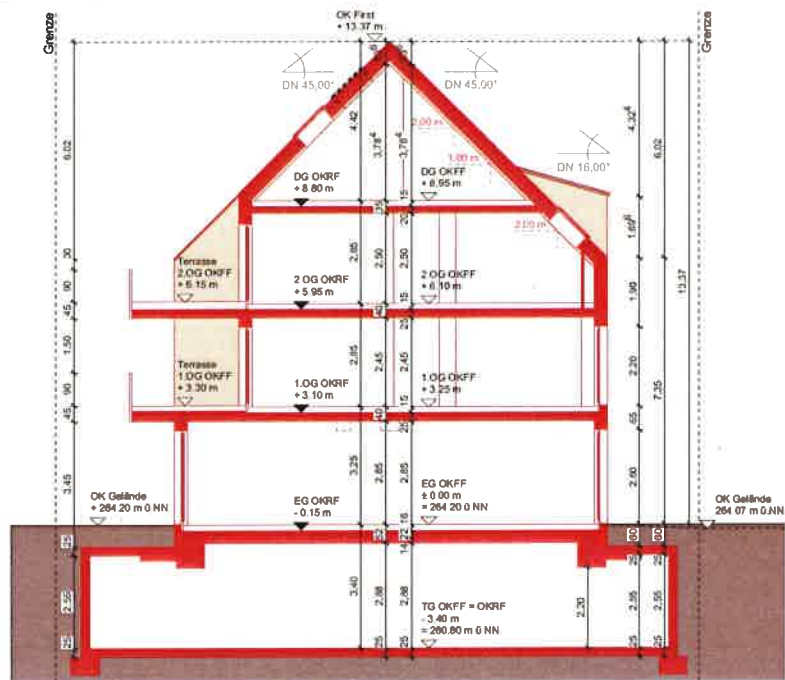
Schnitt B-B
