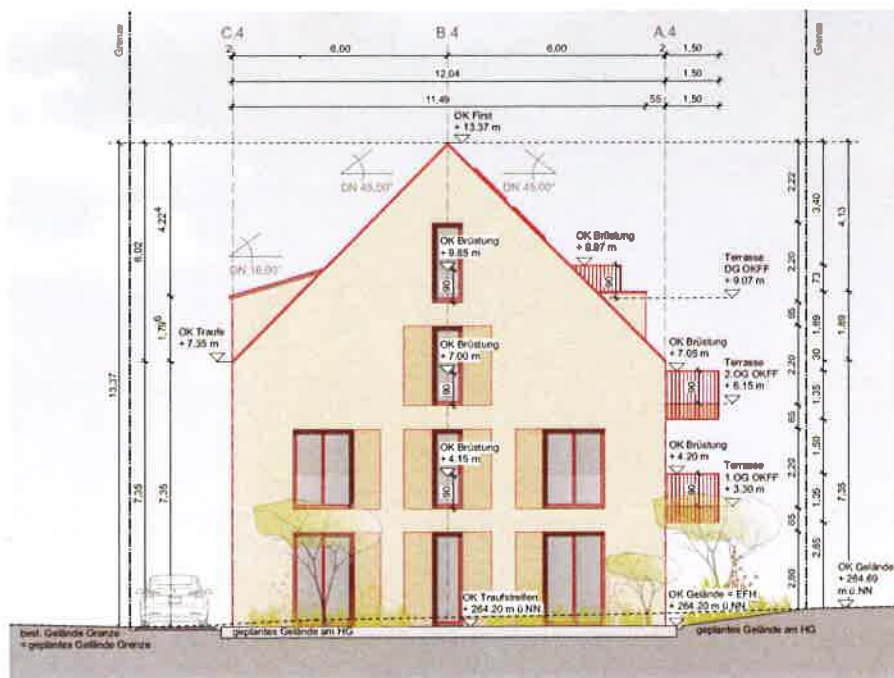
Ansicht Nord 1:100
