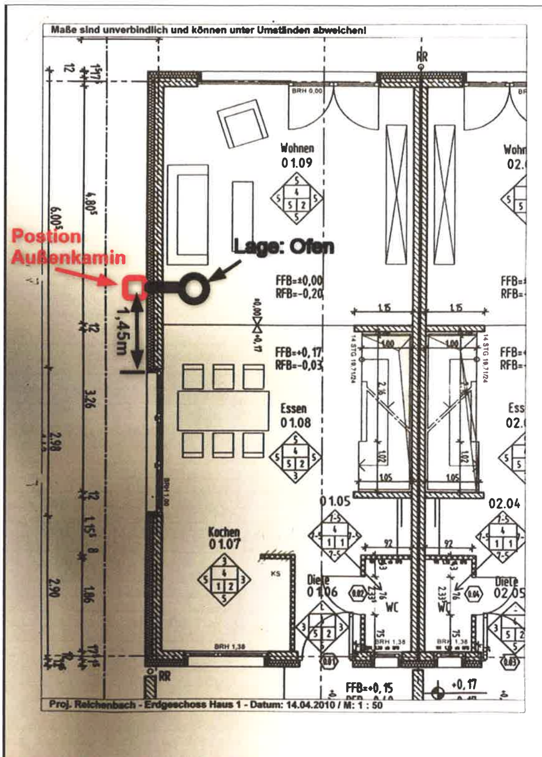
Lageplan 2: Position des Außenkamins Grundriss, Haus Hauptstraße 5/5 ; 73262 Reichenbach
