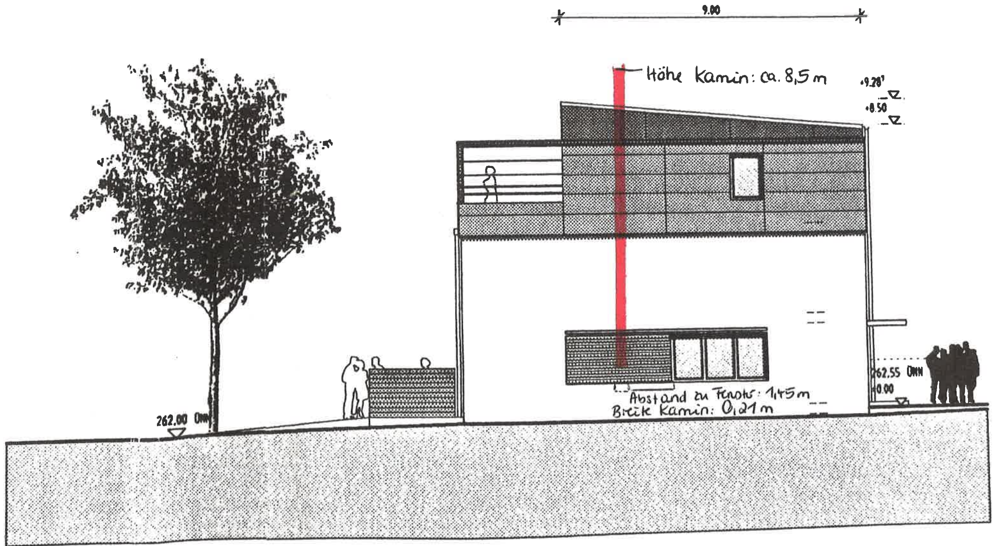
Abb.: Ansicht Giebel Reihenhäuser (Maßstab 1:100)
