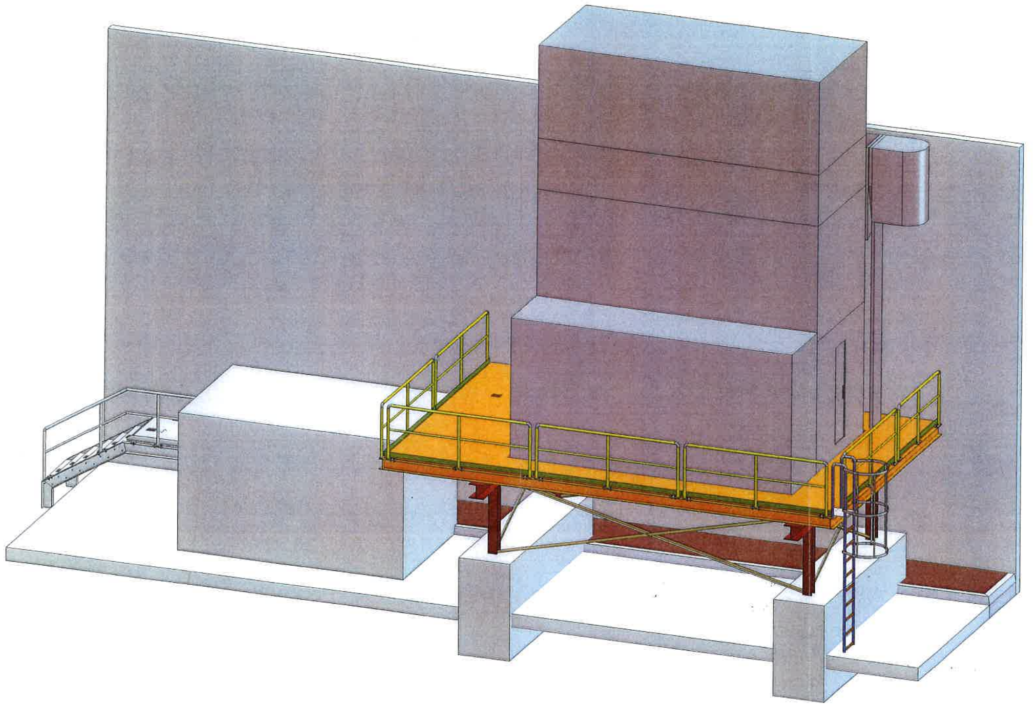
Ansicht Verflüssiger-Aggregat
