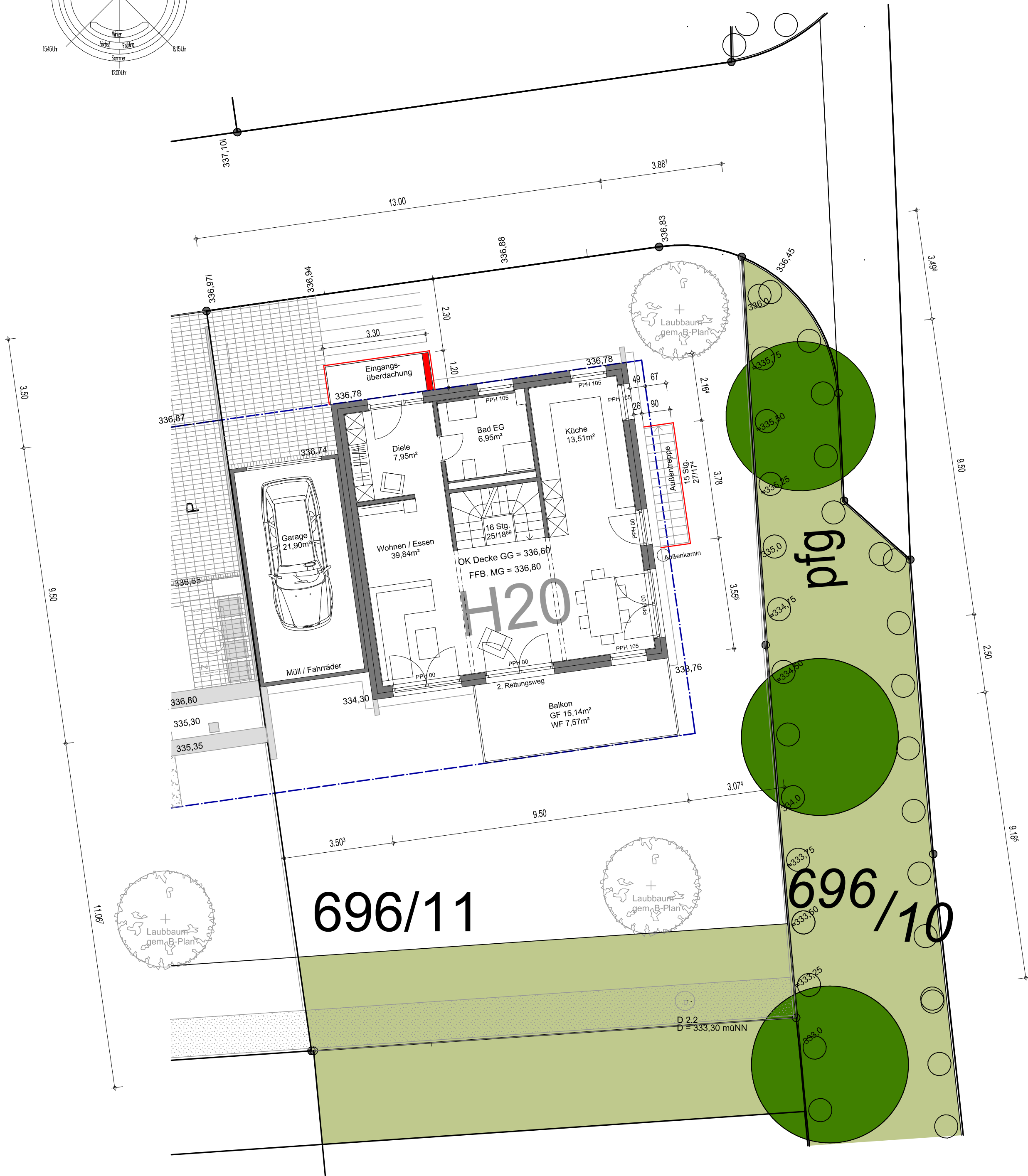
Grundriss Erdgeschoss (Mittelgeschoss MG) im Lageplan M 1/100
