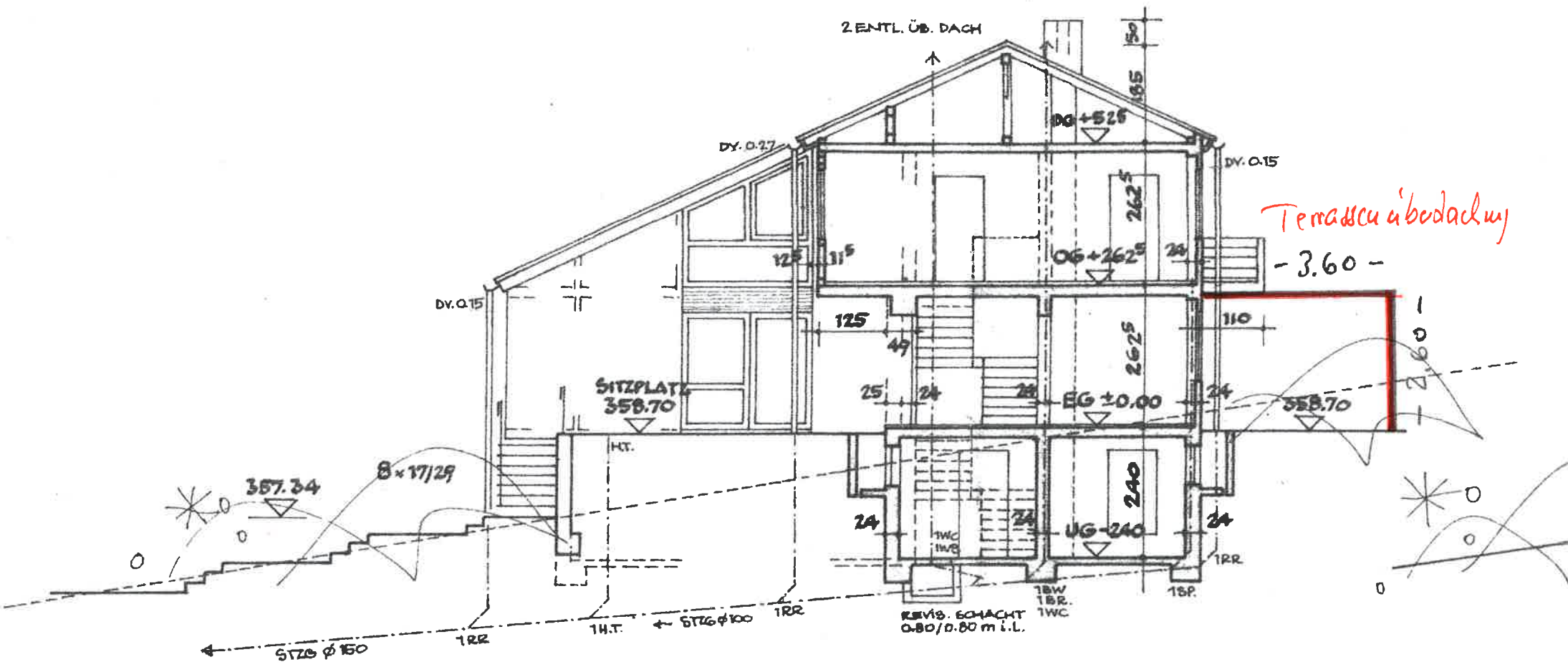
SCHNITT I - I
