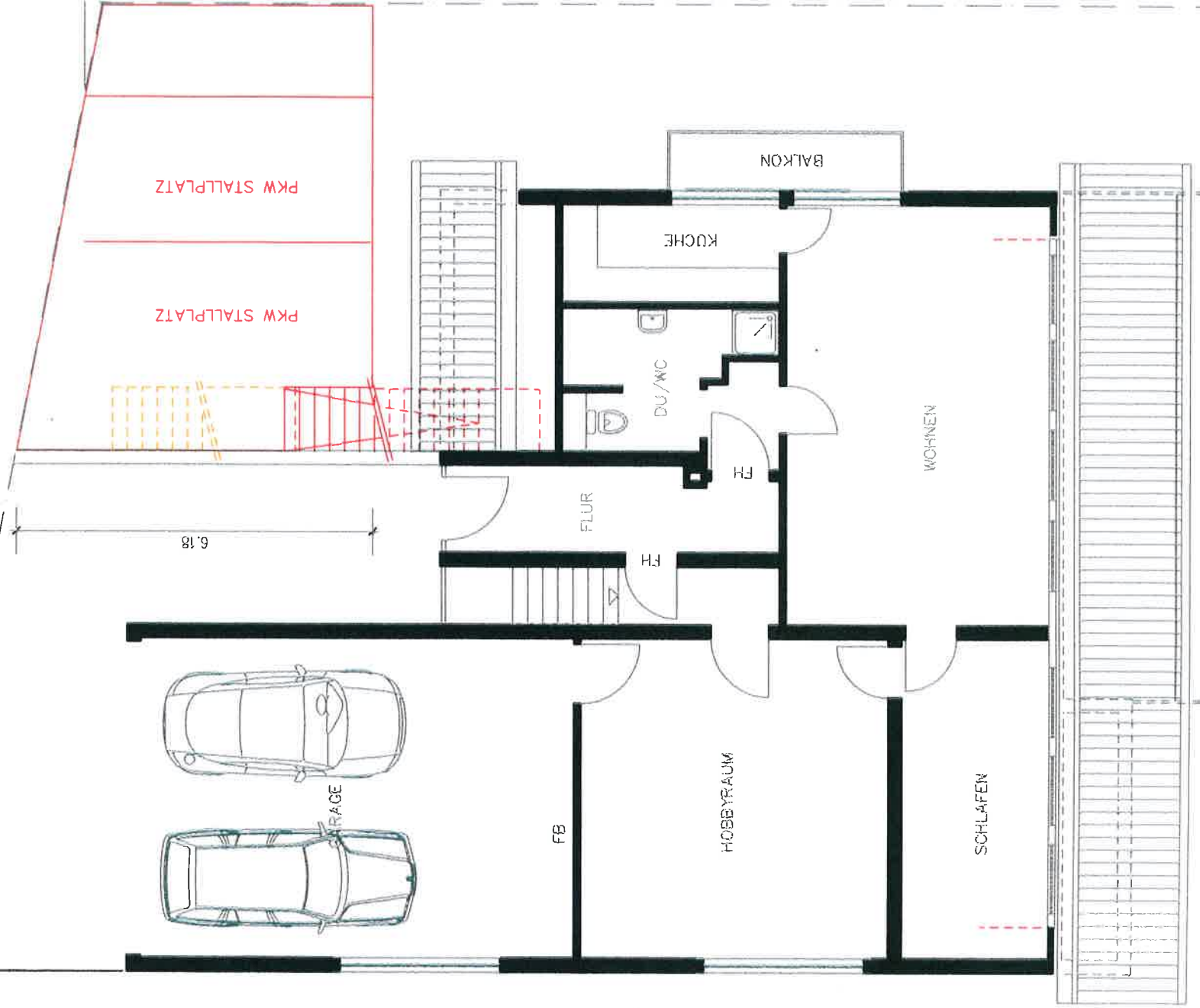
Grundriss 1. Obergeschoss v. 17.05.21 M 1:100
