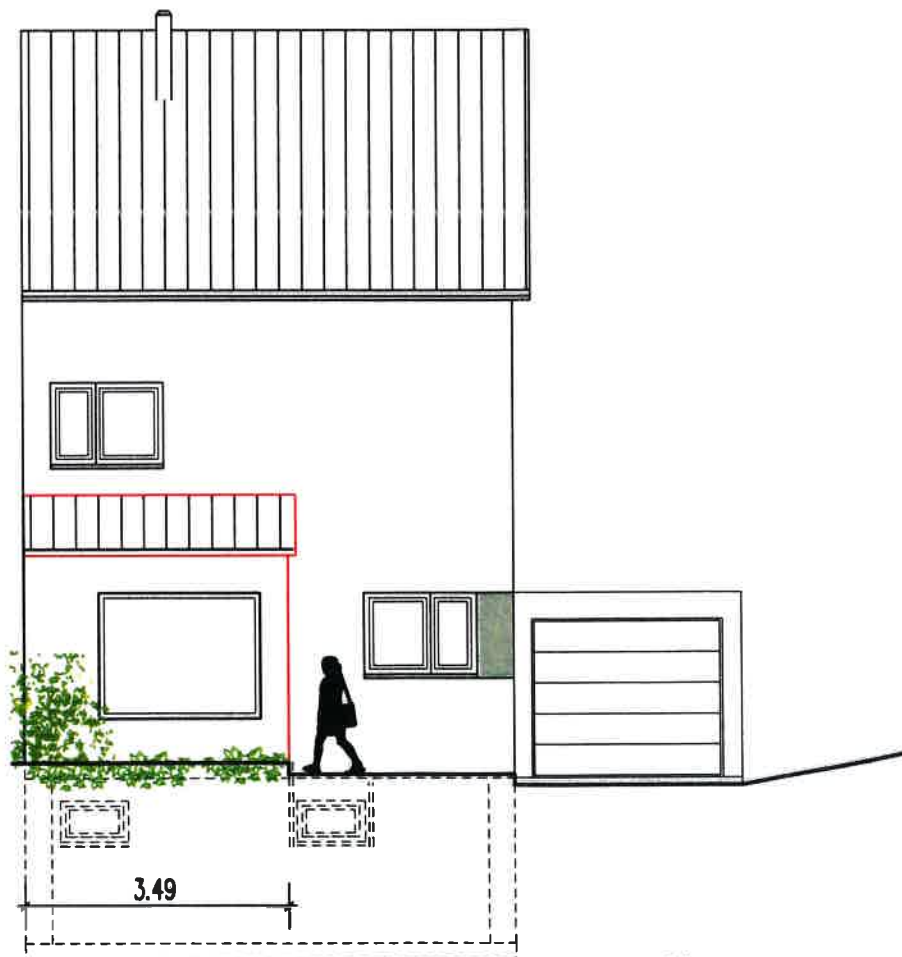
Ansicht Nord
