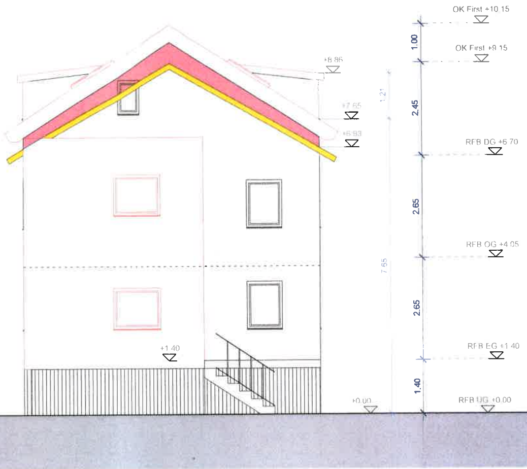
Ansicht Ost
