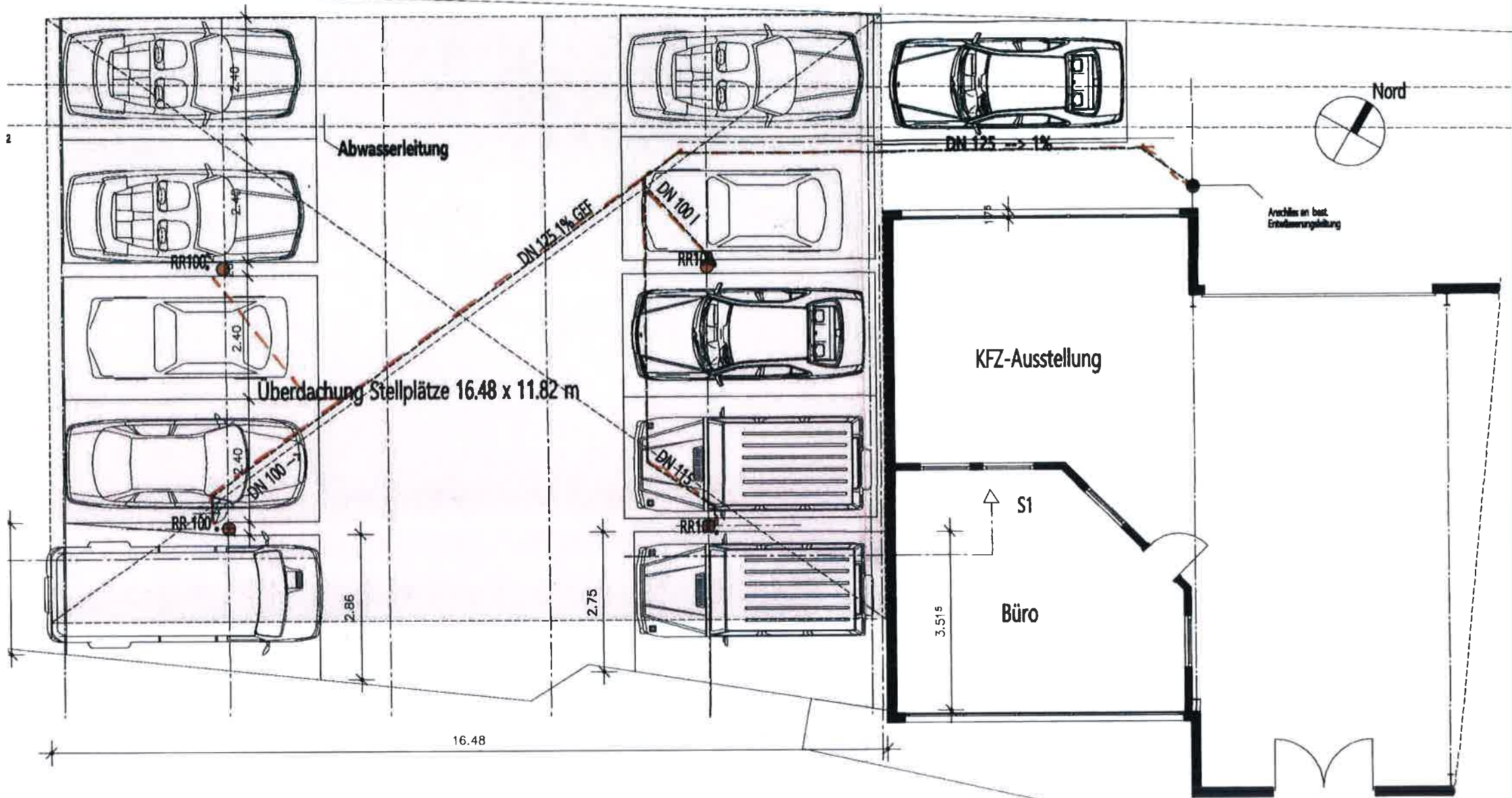
GRUNDRISS ERDGESCHOSS(m. Entwässerung) v. 14.10.2022, M 1:100
