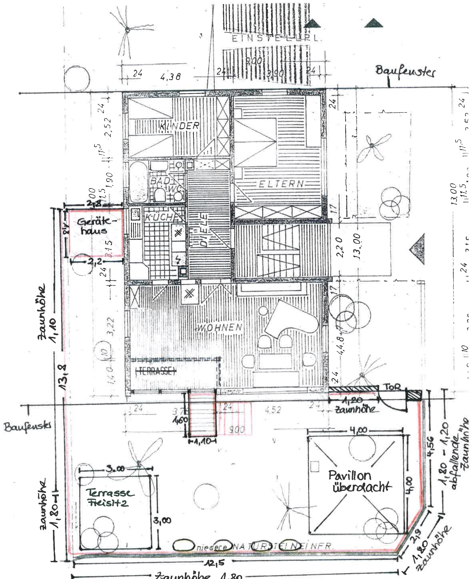
Grundriss EG v. 05.06.2023 M 1 : 100
