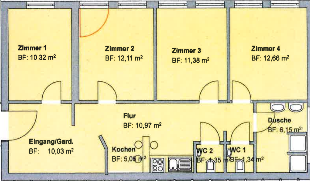
Grundriss EG v. 03.05.2023, M 1:100
