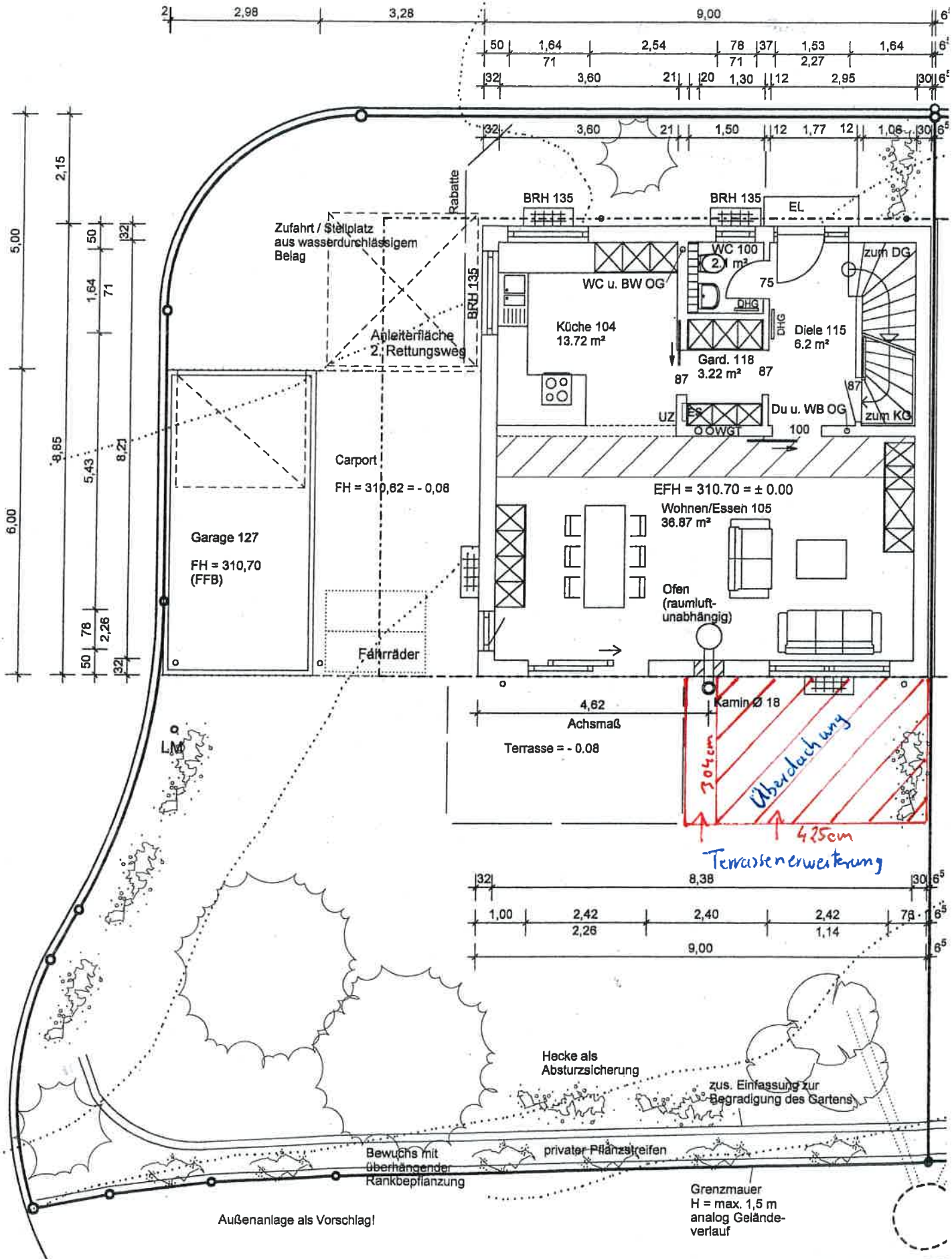
Grundriss EG v. 29.10.2023 M 1:100
