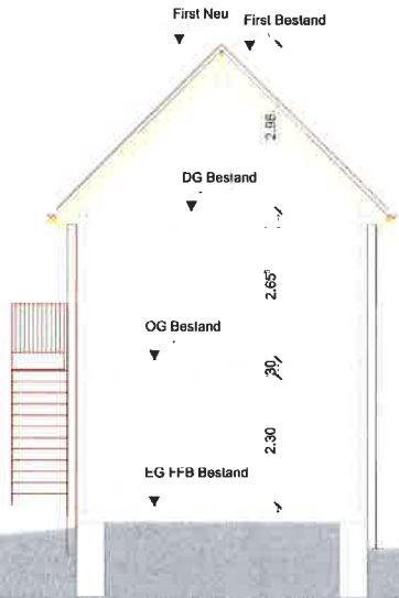
Schnitt A-A
