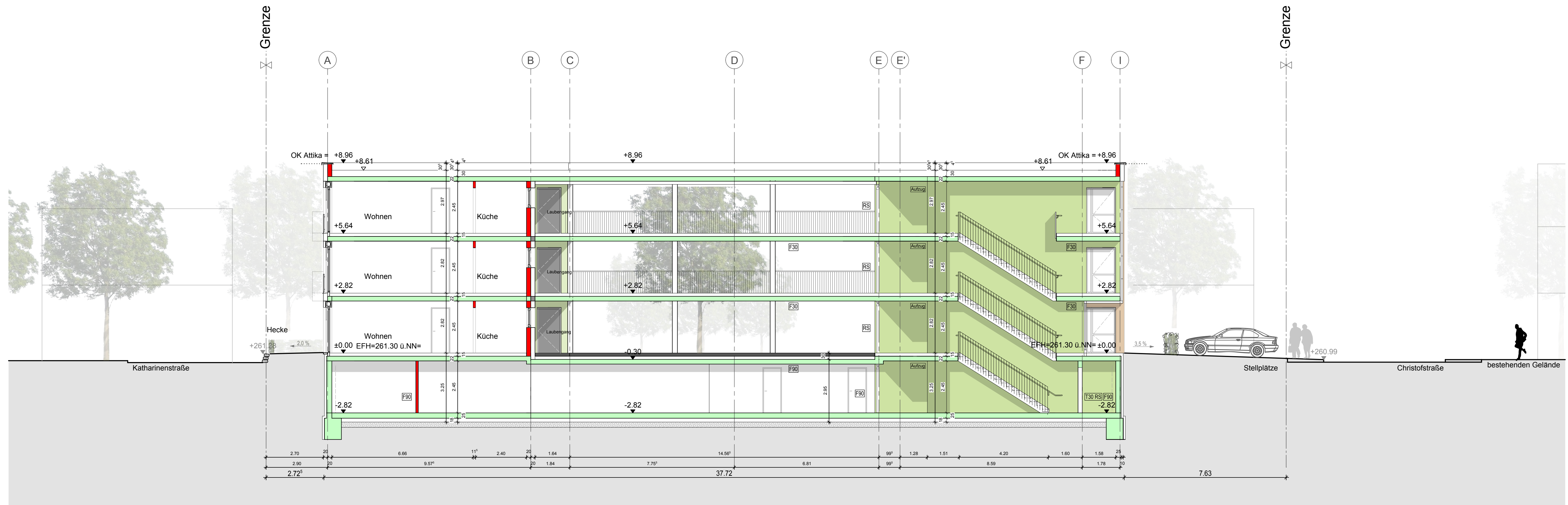
Schnitt C-C M 1:100
