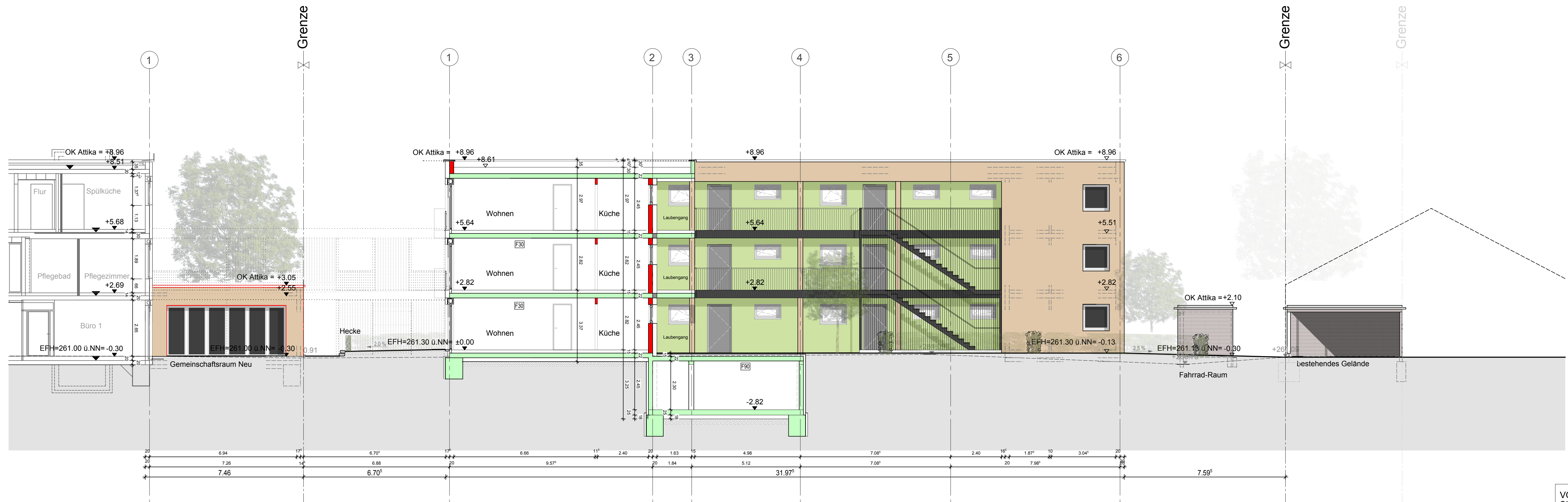
Schnitt B-B M 1:100
