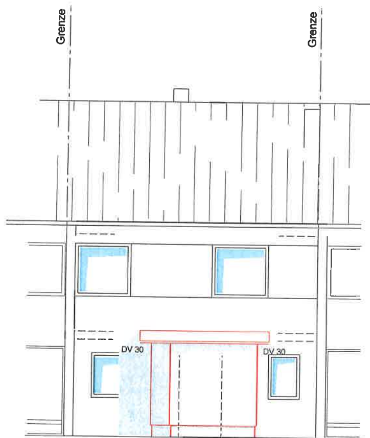
Ansicht Nord
