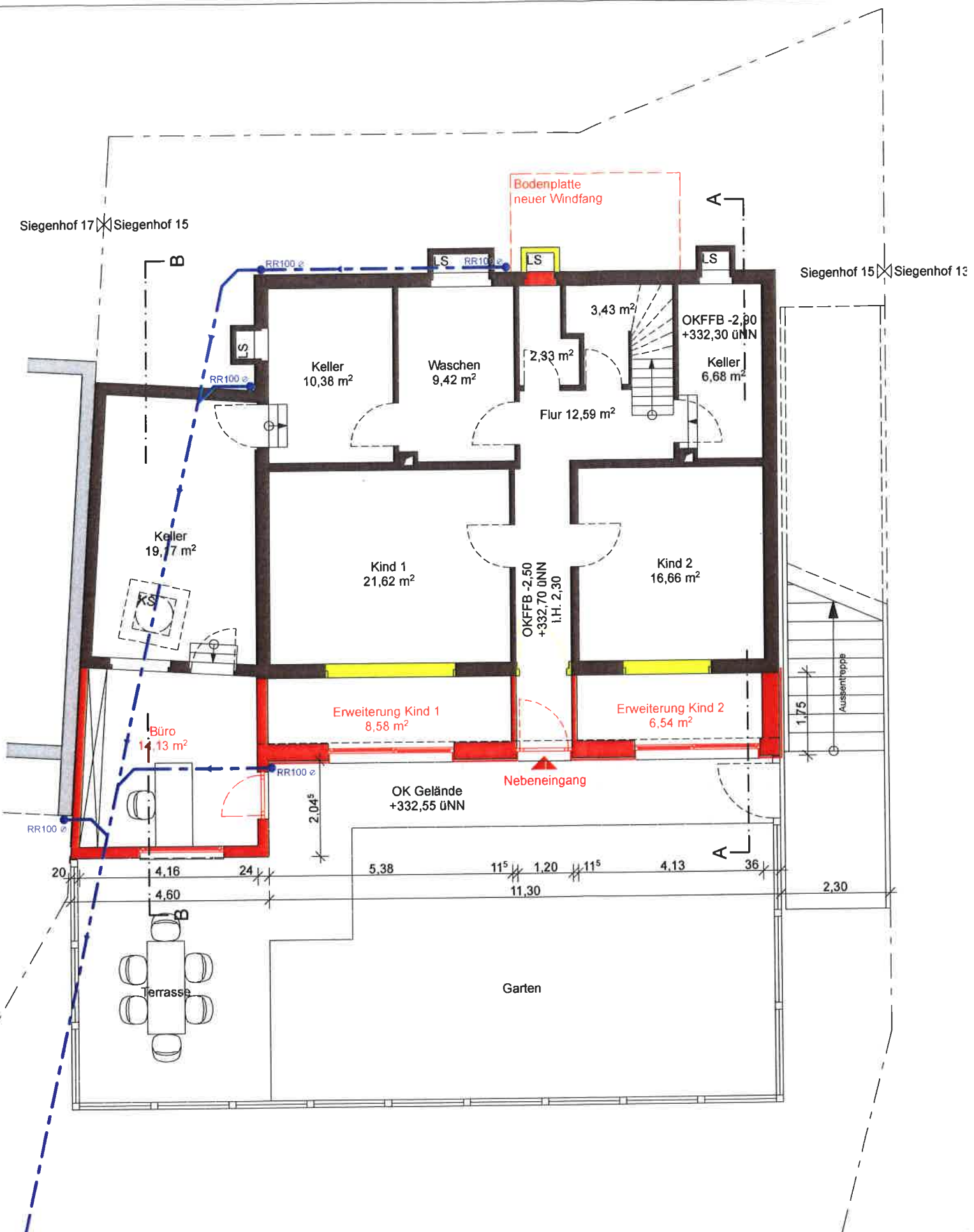
Grundriss UG M 1:100
