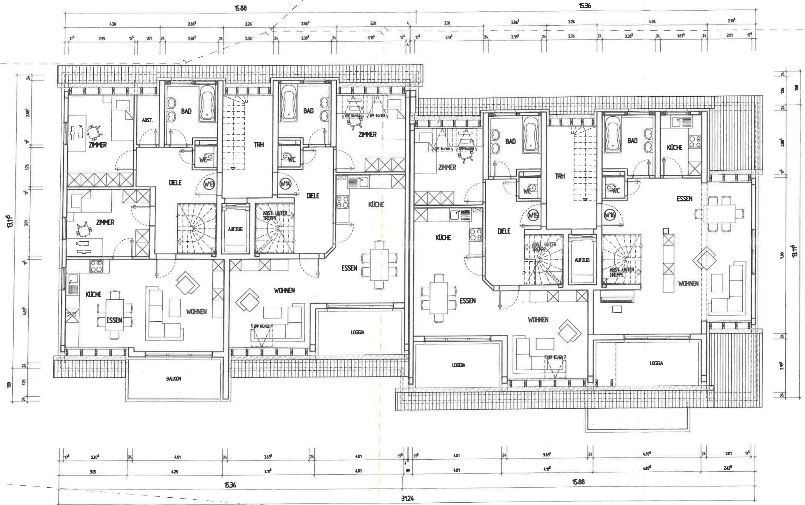
MEHRFAMILIENHAUS REICHENBACH – FILS SEESTRASSE 32/36 GRUNDRISS 1. DG 1:100
