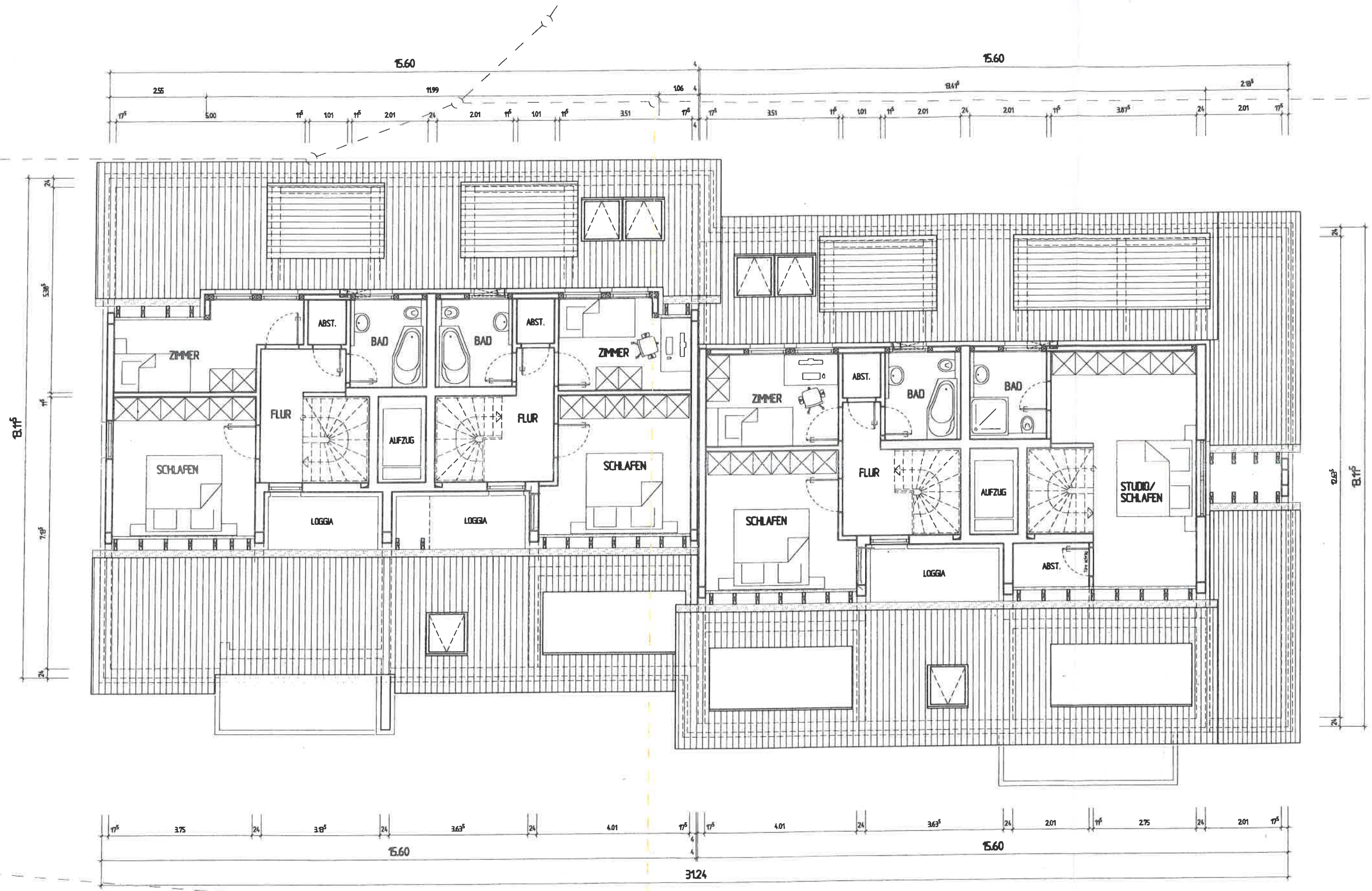
MEHRFAMILIENHAUS REICHENBACH – FILS SEESTRASSE 32/36 GRUNDRISS 2. DG 1 : 100
